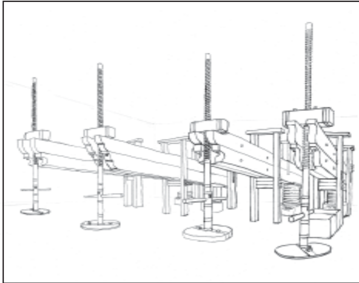
Figura 5 Reconstrucció de les quatre premses del molí. (E. Barrobés)
