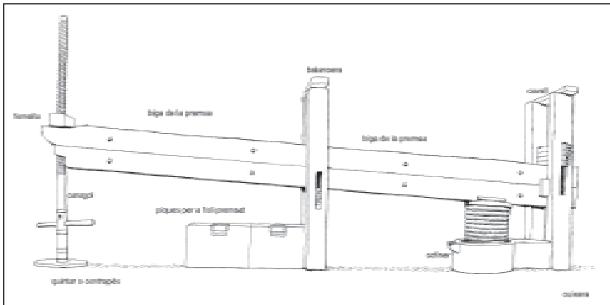
Figura 6 Dibuix d'una premsa de biga tipus. (E. Barrobés)
