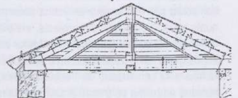
Armadura de la cubierta de la cúpula. (Fig. 5.ª)
