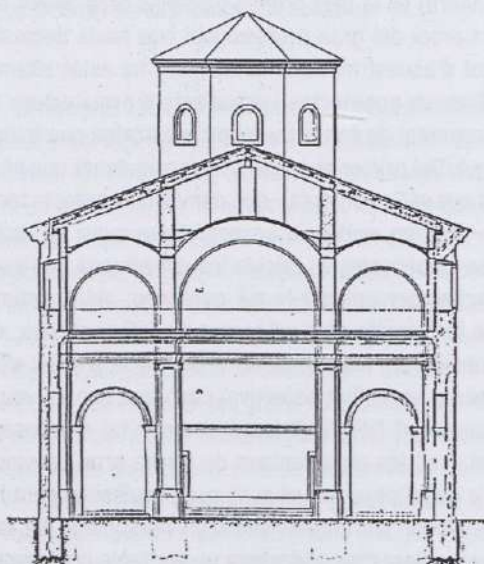
Sección transversal por C-D.
