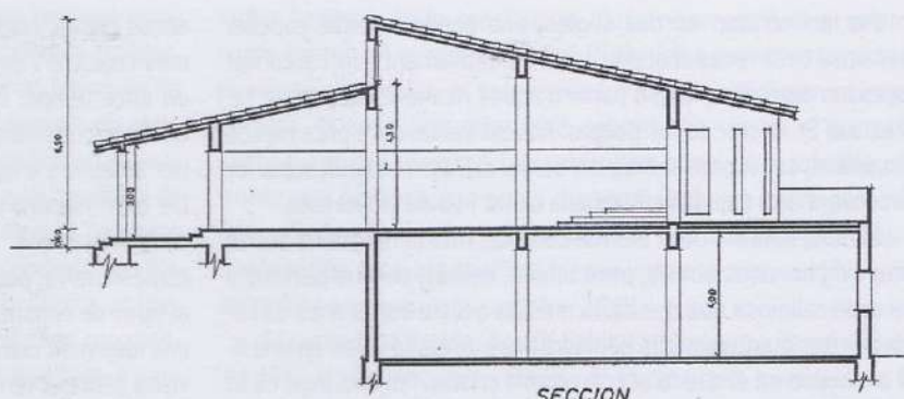
SECCION
