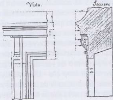
Decoracion de la puerta de entrada. (Fig. 1.ª)
