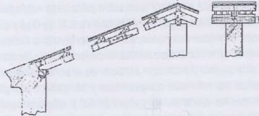
Armadura de la cubierta del templo. (Fig. 4.ª)
