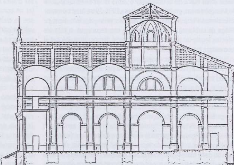
Sección longitudinal por A-B.
