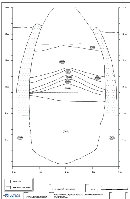
FIGURA 4. Imatges exterior i interior, i secció, de la sitja núm. 2.
