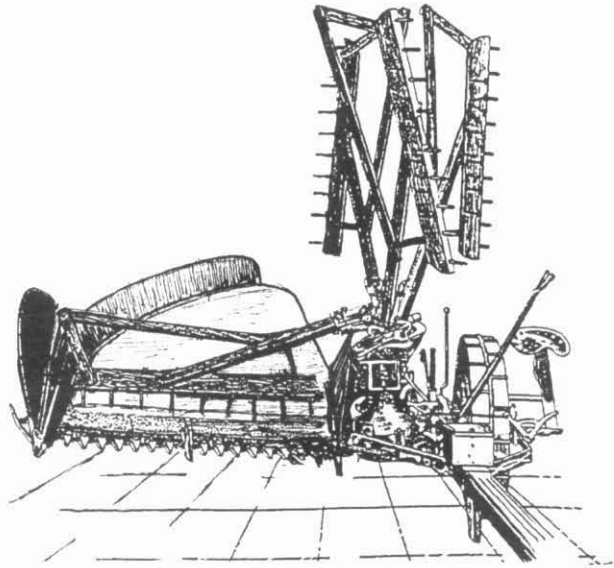
Màquina gavelladora a punt de segar (Dibuix deixat per J. Trepat – Tàrraga)
