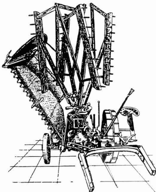
Màquina de segar gavelladora plegada per anar per camins (Dibuix deixat per J. Trepas)
