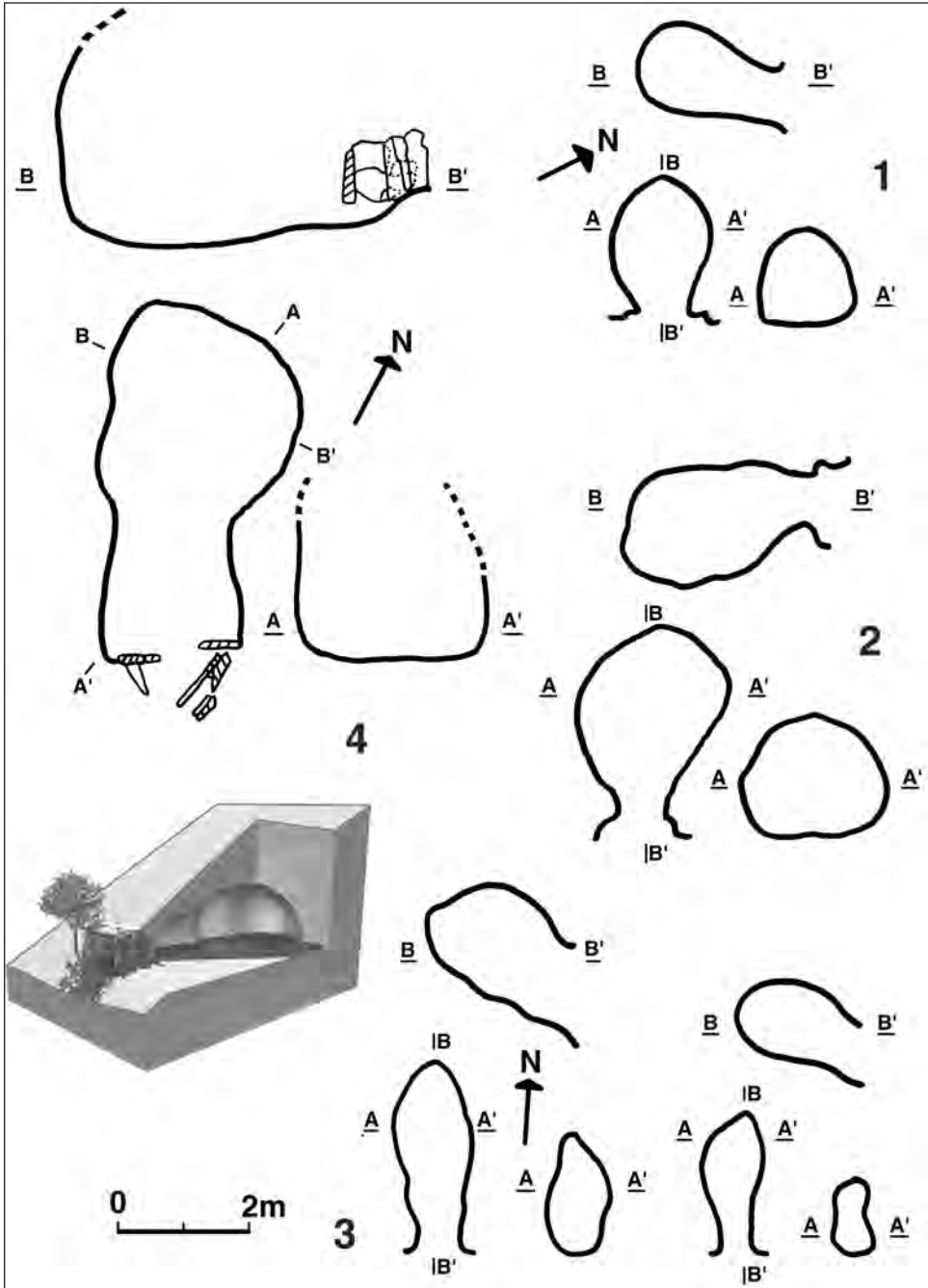
Fig. 2. Plantas de algunos hipogeos catalanes. 1. Mas Rissec (a partir de Tarrús & Chinchilla, 1992), 2. La Tuna (a partir de Esteva, 1958), 3. Ses Falugues I y II (a partir de Berdichewsky, 1964) y 4. Costa de Can Martorell (a partir de Mercadal et Alii , 2003). Todos los hipogeos están a la misma escala excepto la simulación tridimensional de Costa de Can Martorell (de F. Bayés).
