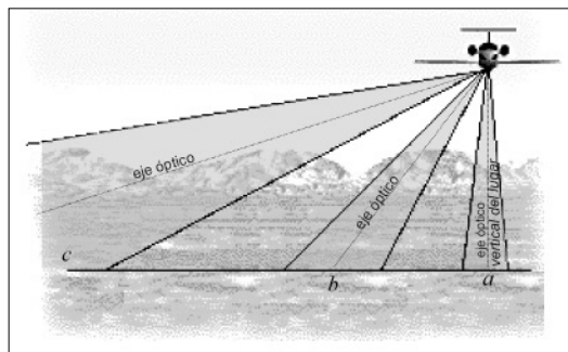
Fig. 2. Diversos tipos de fotografías aéreas según su ángulo de adquisición. a: vertical; b: oblicua; c: panorámica.
