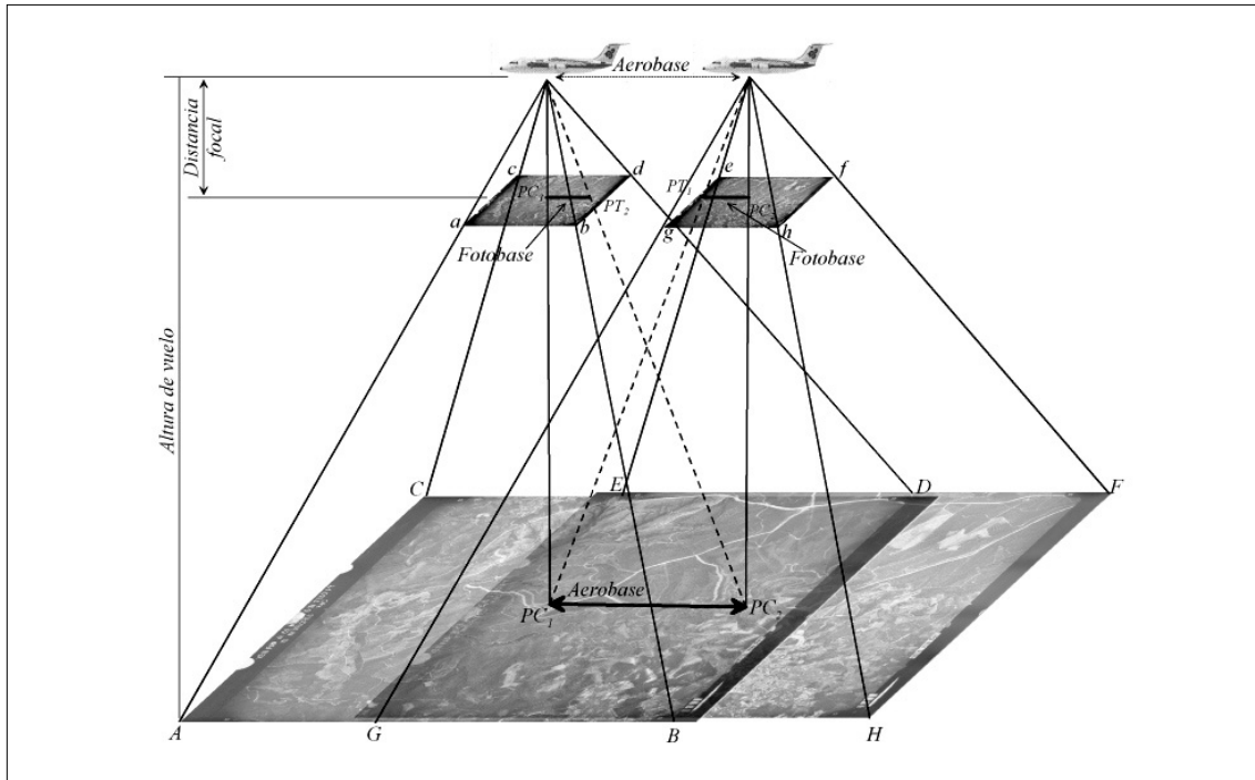
Fig. 5. Adquisición de dos fotografías consecutivas (par estereoscópico). La fotografía de la izquierda abarca el terreno comprendido entre los puntos ABCD, mientras la de la derecha, el comprendido entre EFGH. La área común, EDGB, corresponde a 2/3 del total de terreno fotografiado y será la zona que se podrá reproducir en visión tridimensional. Aerobase es la distancia que hay entre dos tomas sucesivas de fotografías; su equivalente sobre la fotografía es la fotobase (modificado de Vergara, 1978).
