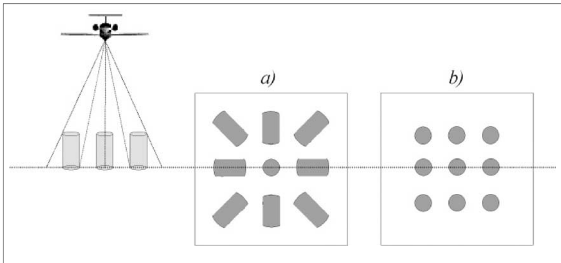
Fig. 4. Desplazamiento radial. Imaginemos nueve cilindros idénticos en una superficie plana, su representación en fotografía aérea es la representada en a), o sea, su desplazamiento es radial a partir del centro de sentido hacia la periferia (proyección cónica); b) proyección ortogonal, o sea, la misma que en los mapas.
