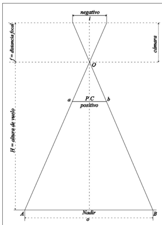
Fig. 3. Terminología de una fotografía vertical. Altura de vuelo ( H ) en el momento de la toma es referida al nivel del mar. Altura de vuelo sobre el terreno ( H_0 ) es la distancia existente entre el centro de la cámara y el terreno en el momento de la exposición. Distancia focal ( f ) es la distancia que existe entre el foco de la lente y el negativo de la película. Eje óptico es la línea ideal que, pasando por el centro de la cámara, es perpendicular a la película expuesta en su punto medio. Punto central (PC) es la intersección del eje óptico y la película; corresponde al centro geométrico de la fotografía. Nadir (N) es la proyección vertical del centro de la cámara sobre el terreno en el momento de la exposición; cuando la fotografía es absolutamente vertical, el nadir coincide con el punto central, es decir, con la proyección del eje óptico. La distancia focal y la altura de vuelo no están a la misma escala (modificado de Lopez Vergara, 1978).
