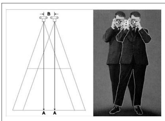
Fig. 6. Toma de pares de fotos estereoscópicas con cámaras de formato pequeño (adaptado de manual del estereoscopio de bolsillo TS 4 de Zeiss).
