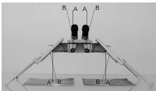
Fig. 8. Estereoscopio de espejos TPOCON MS-3. Si en lugar de enfocar la vista paralela a los ejes ópticos de las lentes, como sería lo correcto (línea AA'), se enfoca al plano de las fotografías, por la costumbre que se tiene de hacerlo así para ver cualquier objeto (línea BB'), la distancia resultante entre B'B' será menor que la AA', lo que obliga a, incorrectamente, acercar las fotografías entre sí.
