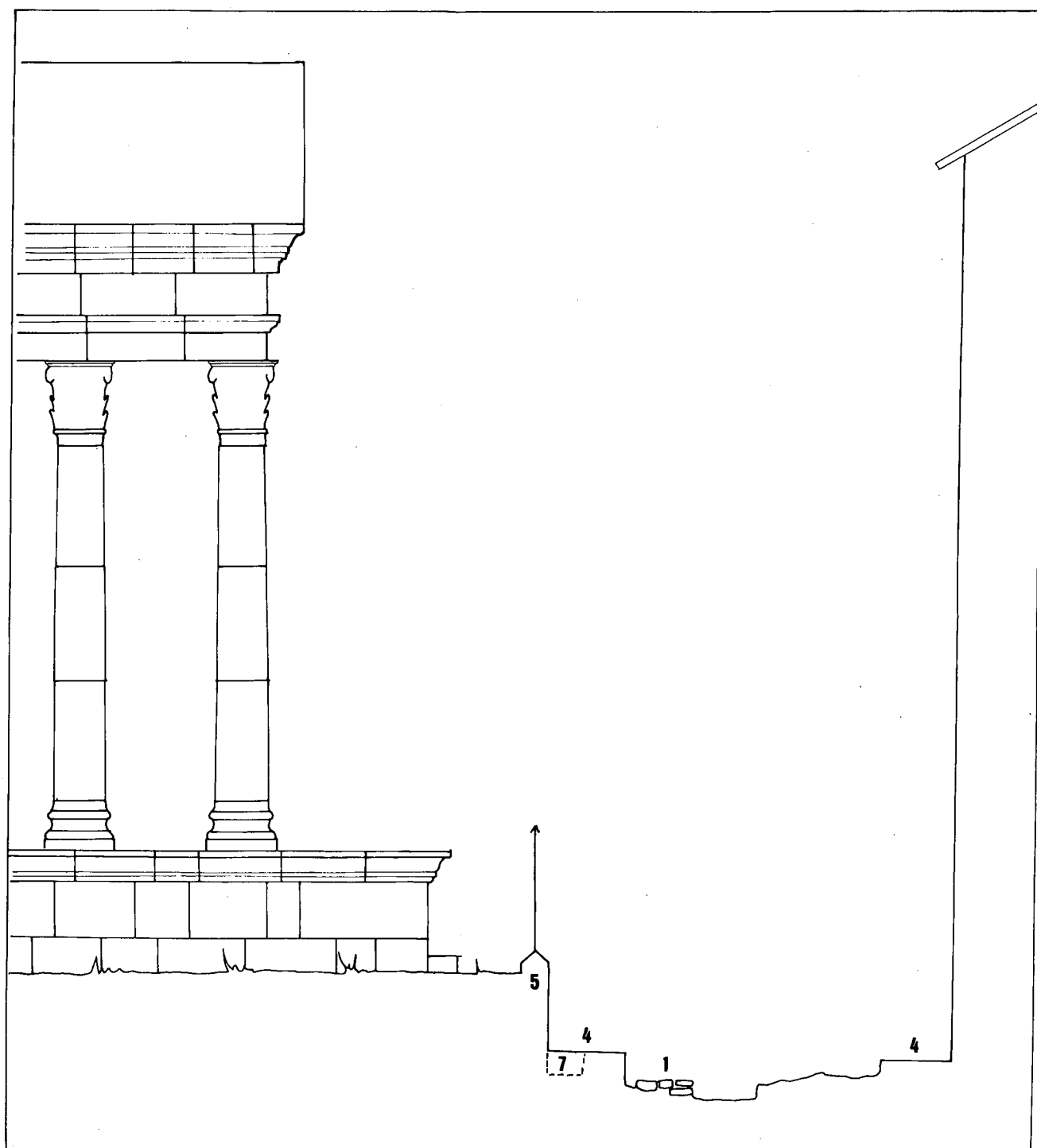
SECCIO' TRANSVERSAL A-A' DEL MUR
