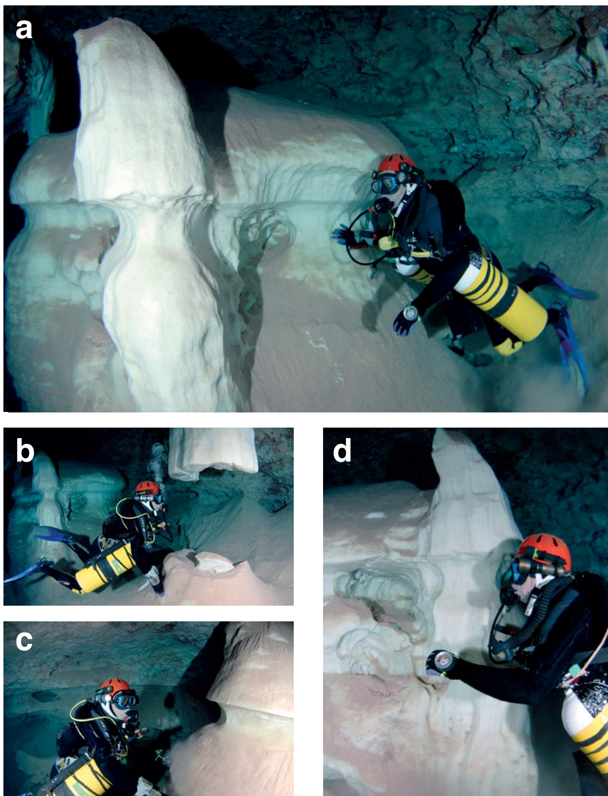
Figura 18: Regata de corrosió ben marcada i molt clara, que es troba a una profunditat sota l'actual nivell freàtic entre -13,5 m i -14 m a una de les galeries de les Haloclines (sector de Ponent). a) Ha afectat, entre d'altres espeleotemes, un gran massís estalagmític, envoltat per aquest solc perfecte. b) Vàries columnes han estat seccionades per la dissolució de l'aigua a l'alçada d'aquesta regata. c) Interessa per igual a la roca mare de les parets i als espeleotemes. d) Està associada a la gènesi d'alguns tupins i galeries iniciadores. (Fotos C. Bodi).
