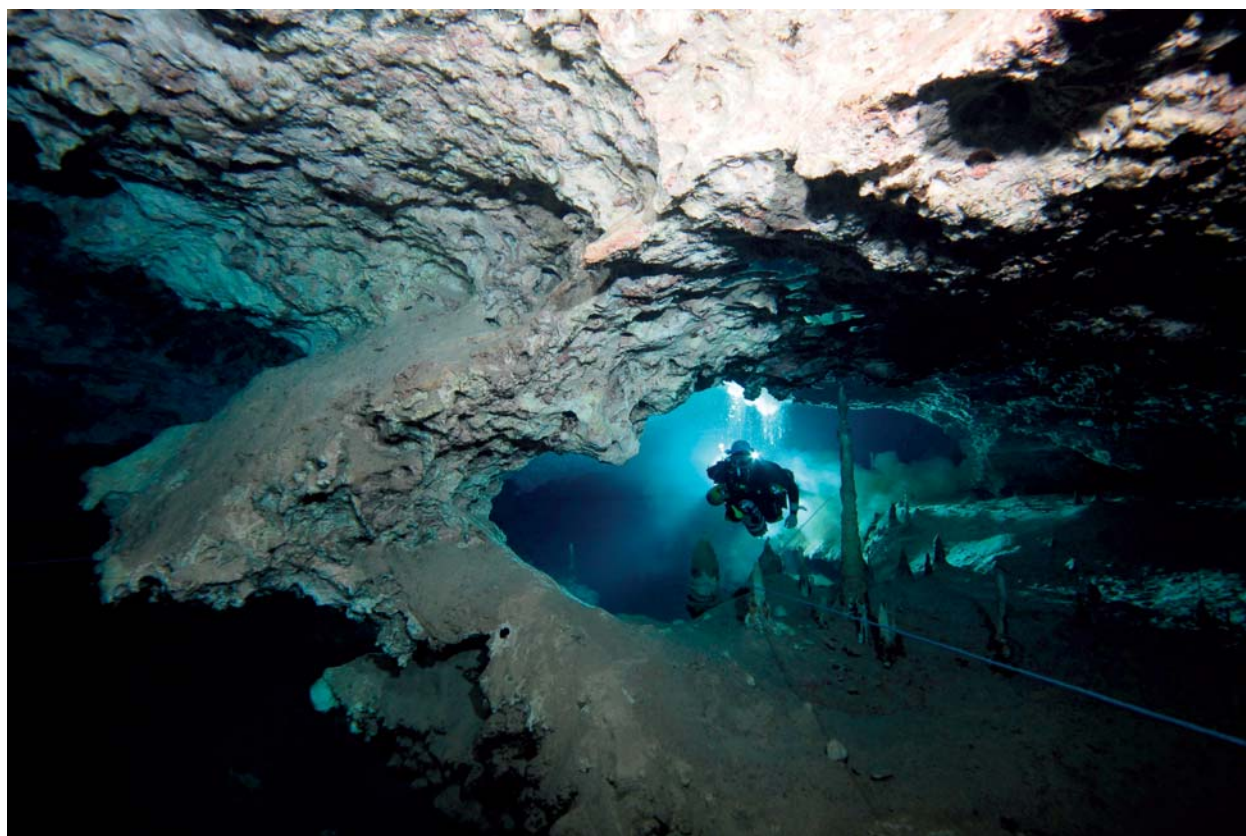
Figura 14: Darrers vestigis d'una galeria freàtica de secció el·líptica al circuit dels Pirates, en haver-se dissolt quasi per complet l'en- và de separació i afegir-se a un àmbit major (Foto C. Bodi).
