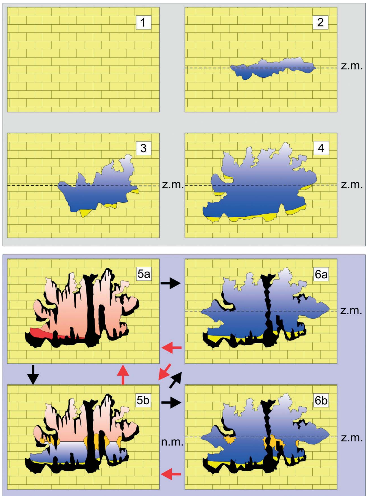
Figura 9: Simplificació dels estadis evolutius d'una galeria freàtica. 1- Acció de la zona de mescla d'aigües sobre la roca calcària. 2-Formació dels primers espais buits i galeries iniciadores. 3-Increment del volum i de les morfologies de corrosió en avançar els processos de dissolució. 4-Acumulació de sediments autòctons carbonatats al terra de la galeria. 5-Davallada del nivell freàtic i evolució de la galeria en condicions vadozes amb la formació d'espeleotemes. 6-Pujada glacioeustàtica del nivell freàtic. Reactivació dels processos de dissolució de la roca i dels espeleotemes, amb la superposició de noves formes primàries.
