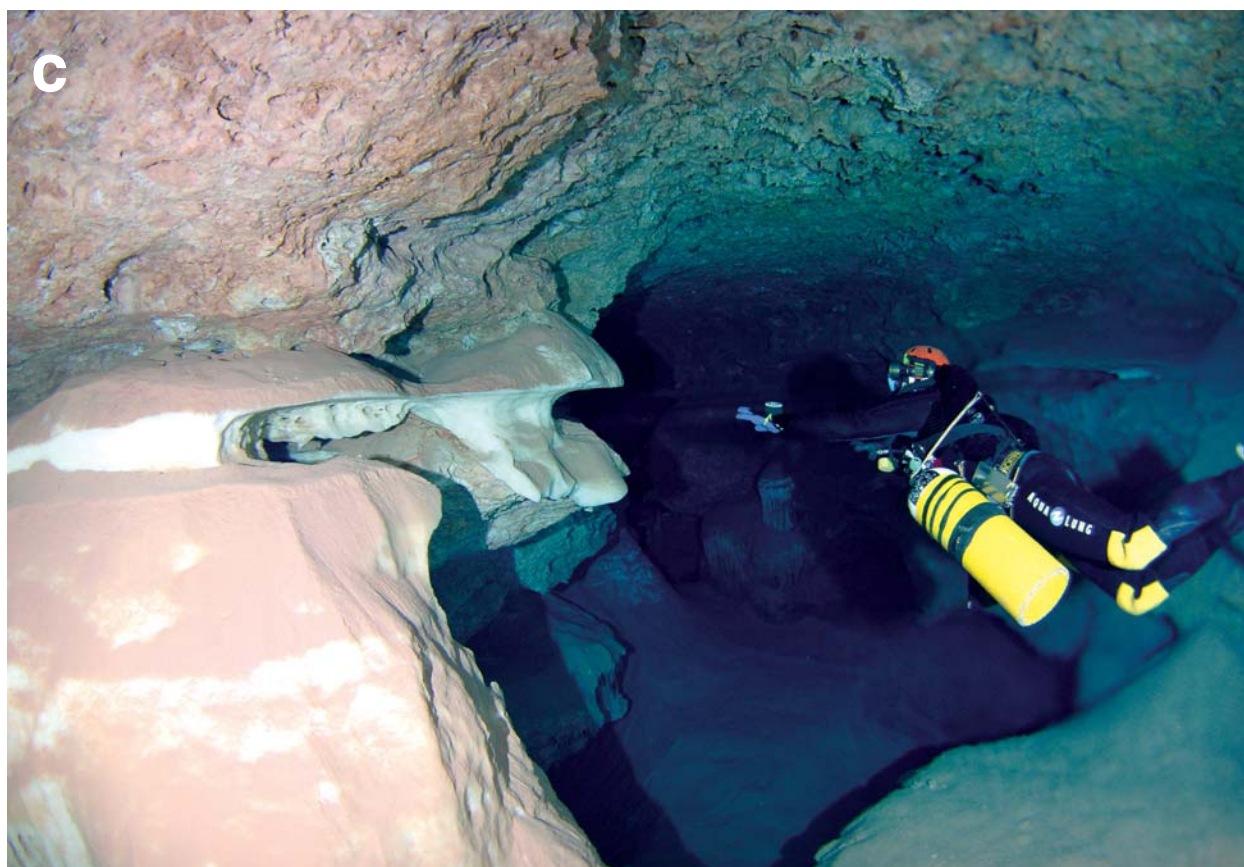
Figura 20: a) Columna tallada a la mateixa cota (-13,5 m) que les morfologies de la Figura 18. b) La regata a una de les parets. c) El solc es manté perfectament definit al llarg de més de 150 m de galeria. (Fotos C. Bodi).
