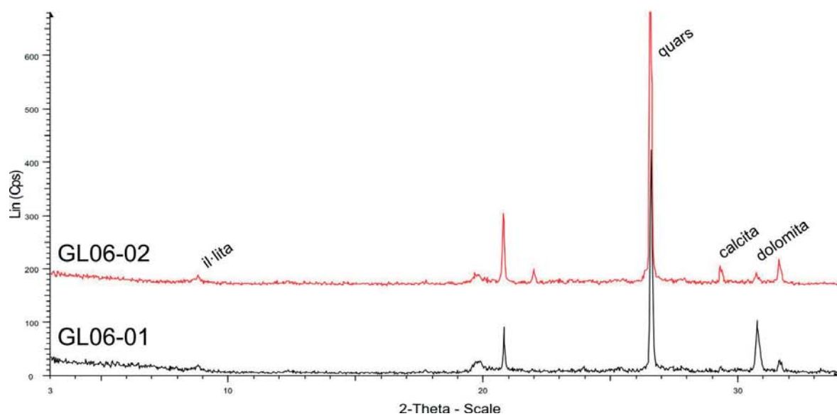
Figura 35: La ciclicitat en la sedimentació és un fet corrent en l'acumulació sedimentària a la cova de sa Gleda.
