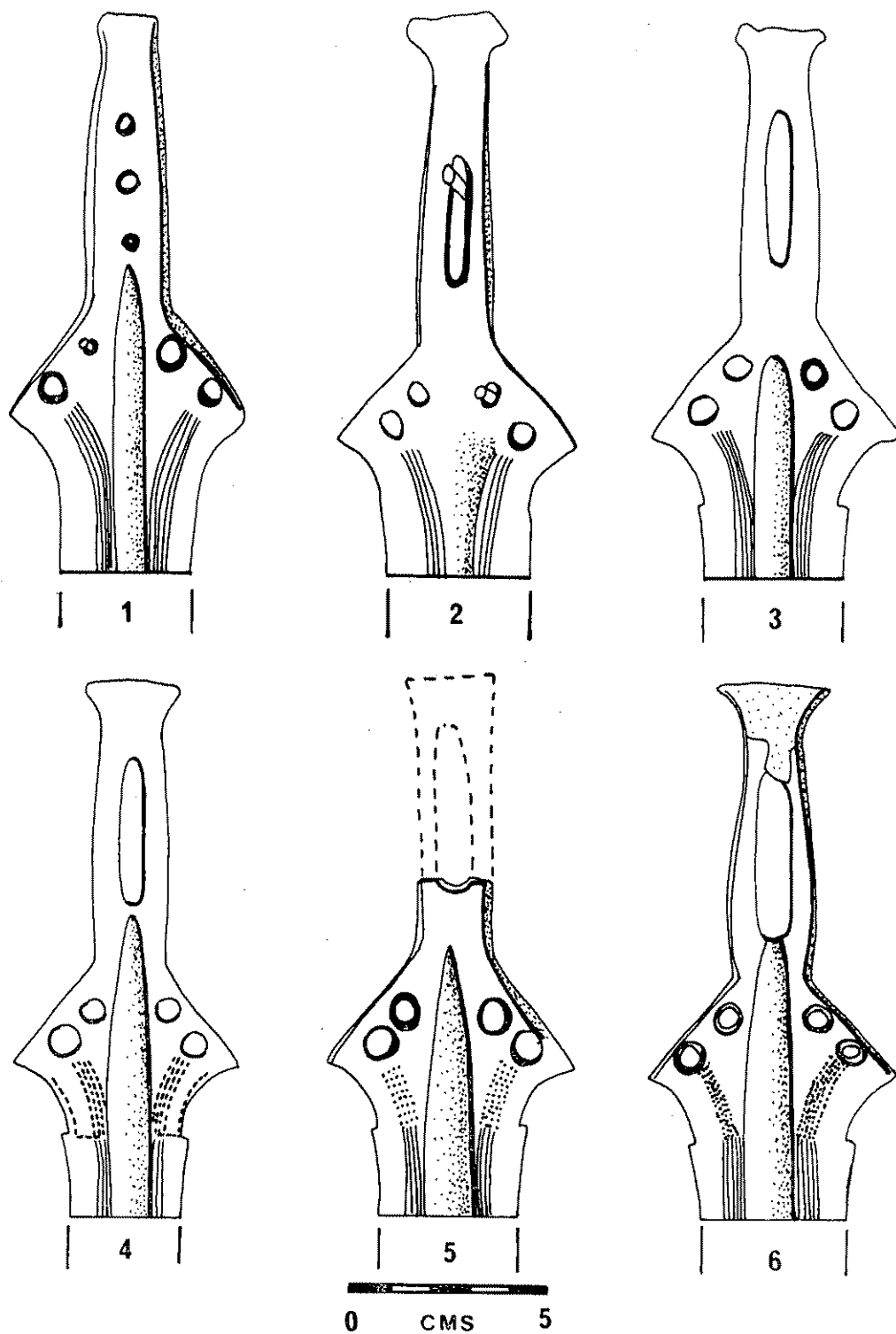
Fig. 2. — [Según Briard, 1965, figs. 63-64]. 1-3, espadas pistiliformes de la región Nantaise con un ricasso débil; 4-6, espadas de la región Nantaise con un ricasso fuerte; tipo de Saint-Nazaire . 1, Bassin de Penhoët, St. Nazaire, L-A; 2, Montoir, L-A; 3, Loire en Nantes, L-A; 4, La Chesine, Nantes, L-A; 5, Nantes, L-A; 6, Montoir, L-A.
