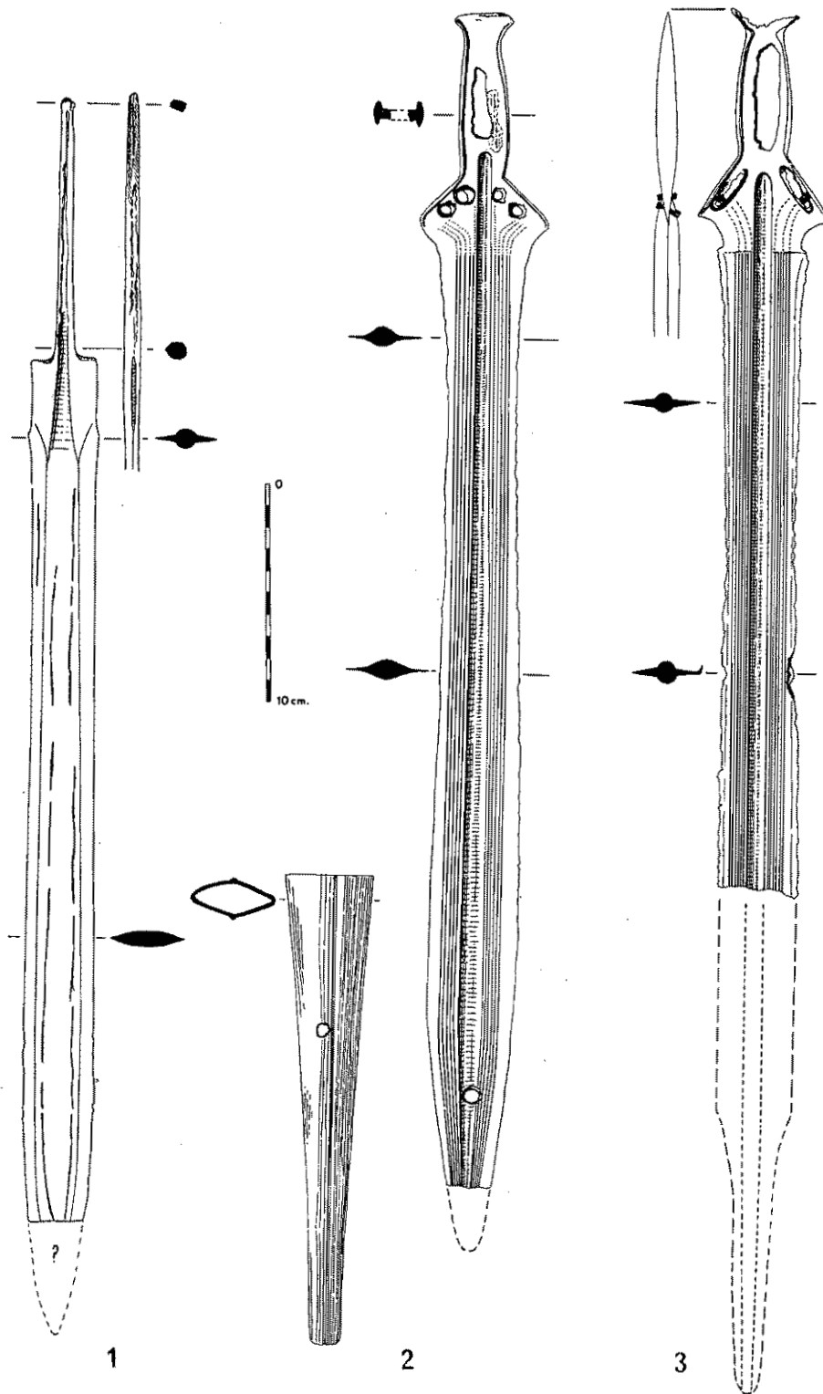
Fig. 1. — 1, espada de Carcabuey, Córdoba; 2, espada de Alhama de Aragón, Zaragoza, con su vaina; 3, espada de Tabernas, Almería.
