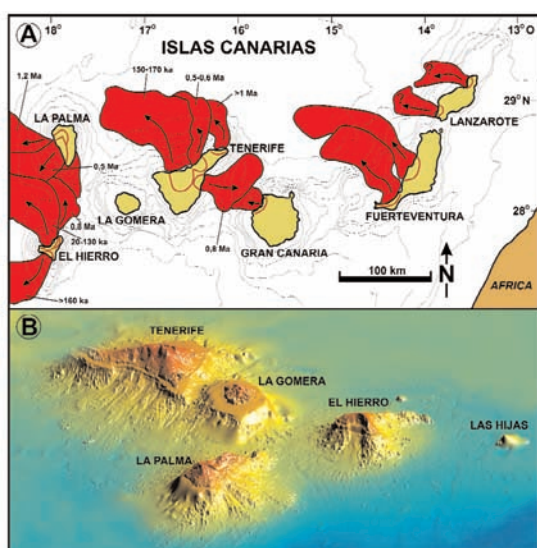
Fig. 5. A. Deslizamientos laterales gigantes en las Islas Canarias (los números indican las edades estimadas de los deslizamientos. Datos tomados de Carracedo, 1994; Urgeles et al., 1999 y Masson et al., 2002). B. Imagen de sonar de las islas occidentales en la que se aprecian claramente los depósitos de avalancha de las islas de Tenerife, La Palma y El Hierro cubriendo los fondos marinos. Obsérvense los volcanes submarinos de Las Hijas, que tal vez puedan constituir en un futuro geológico nuevas islas del Archipiélago Canario (modificado de Masson et al., 2002).
