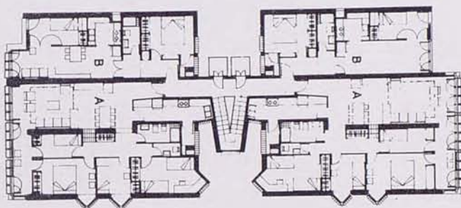
Planta tipo
