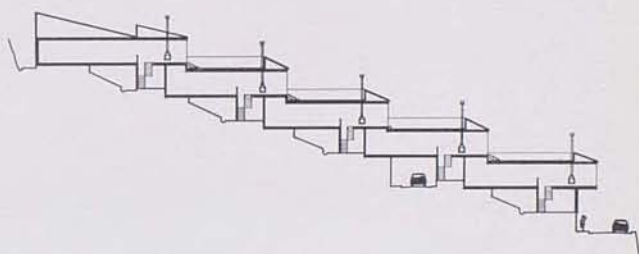
Sección
