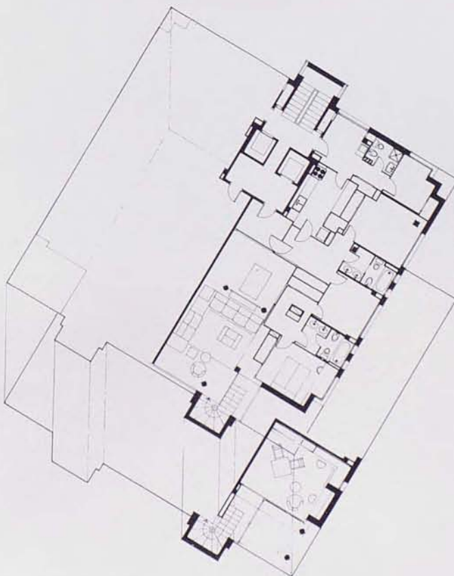
Plantas viviendas duplex
