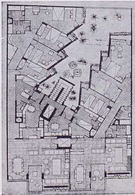
Planta tipo
