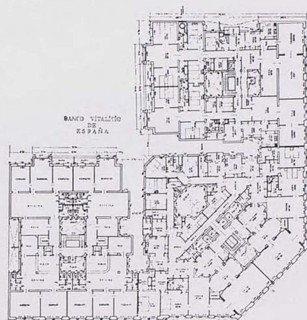
Planta tipo 1.º al 5.º
