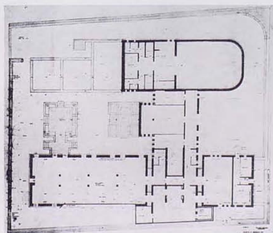
Planta semisótano
