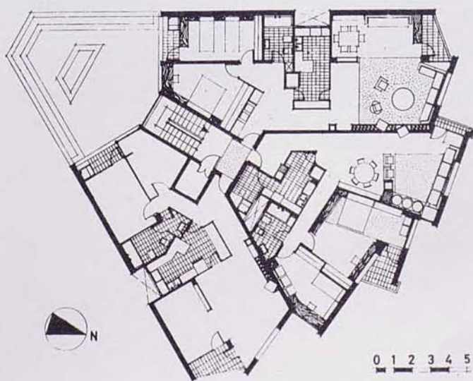
Planta pisos tipo
