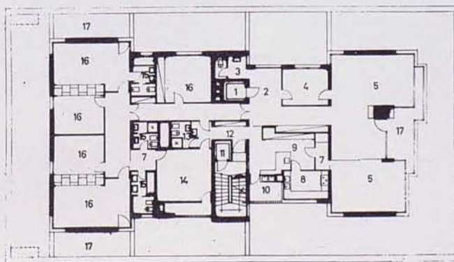
Planta tipo
