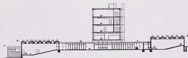
Sección
