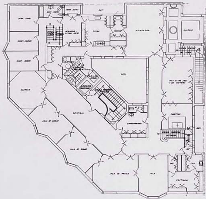
Planta 7.ª
