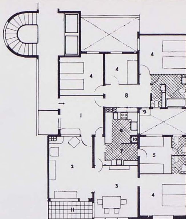
Planta vivienda tipo
