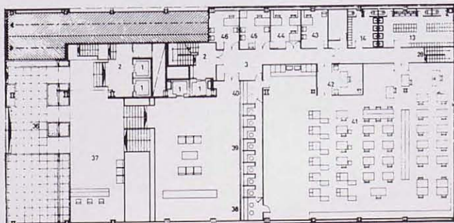
Planta baja
