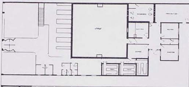
Planta baja
