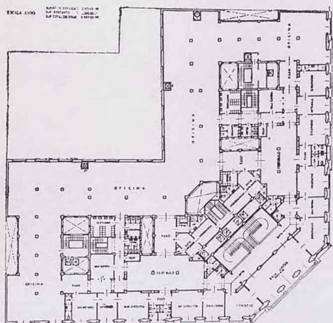
Planta baja
