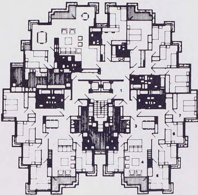
Planta tipo
