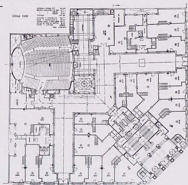
Planta principal
