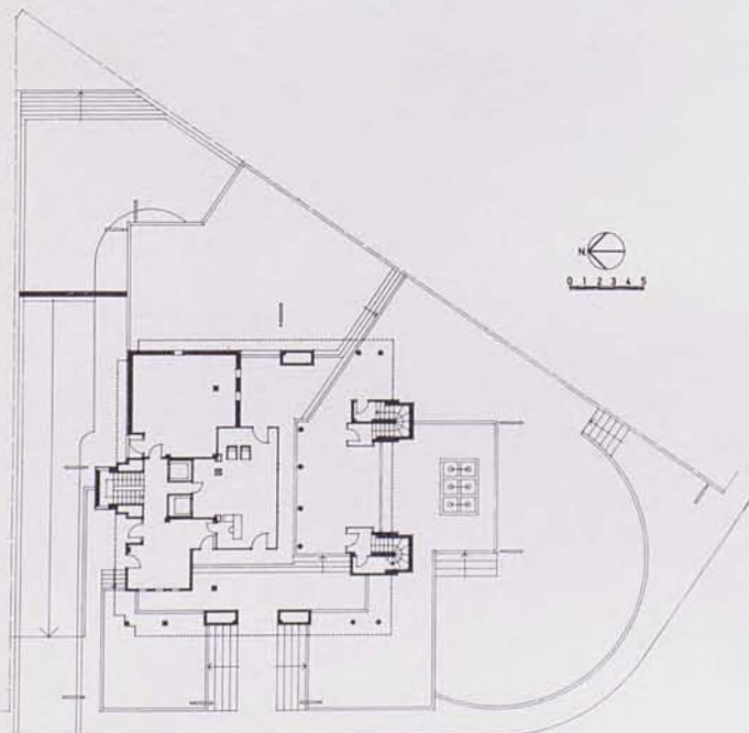
Planta baja
