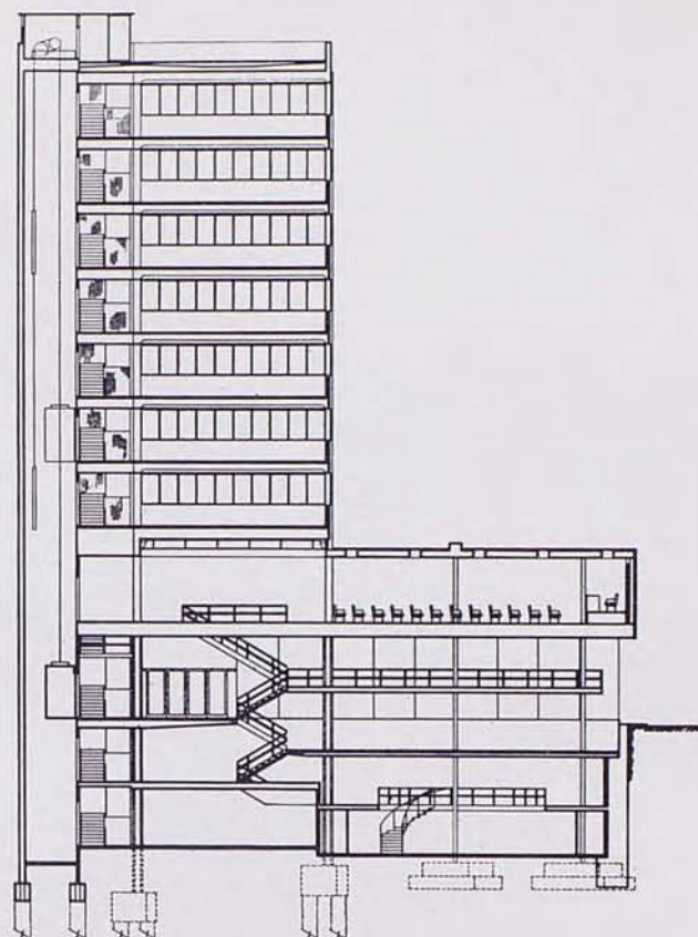
Sección
