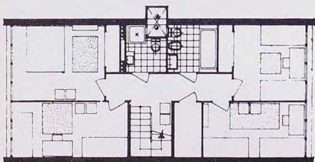
Planta viviendas tipo del bloque C
