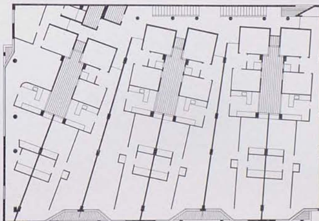
Planta viviendas tipo
