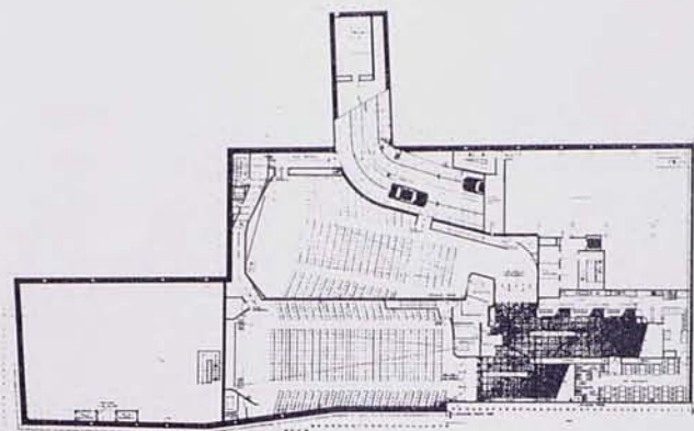
Planta 1.º sótano
