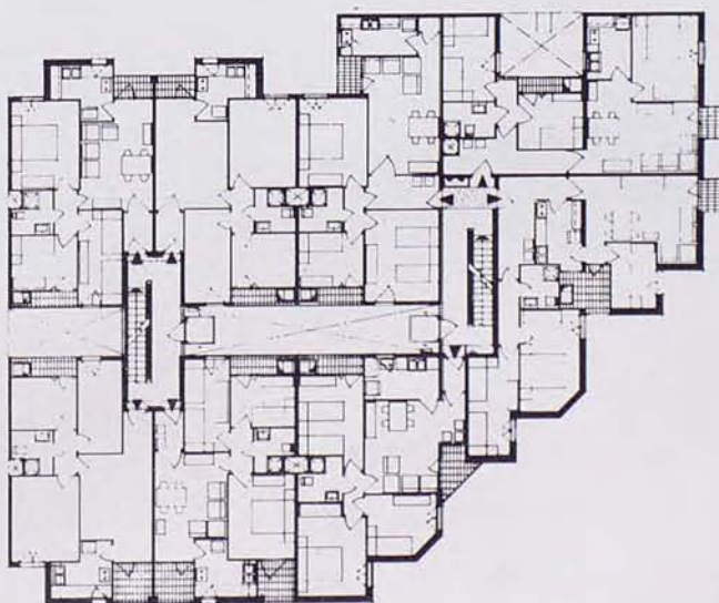
Planta pisos tipo
