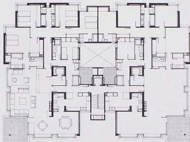
Planta tipo
