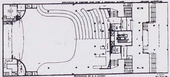
Planta entresuelo-Anfiteatro cine
