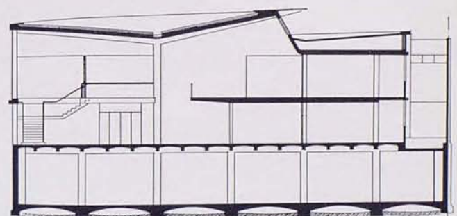
Sección transversal
