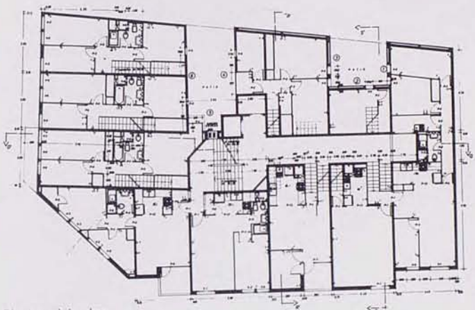
Plantas viviendas
