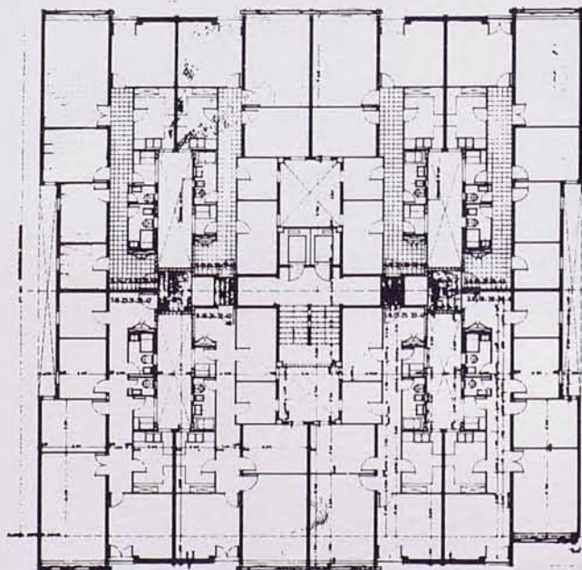
Planta tipo
