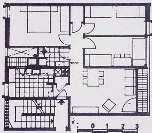
Plano vivienda tipo edificio B
