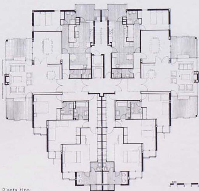
Planta tipo
