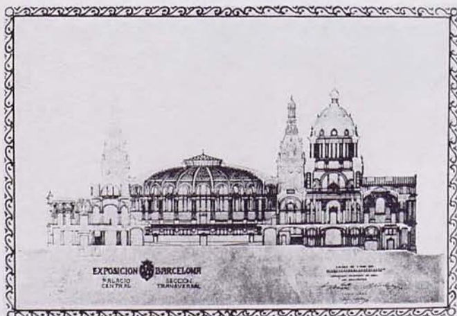
Sección transversal
