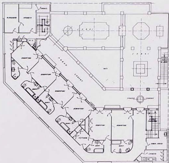
Planta 8.ª
