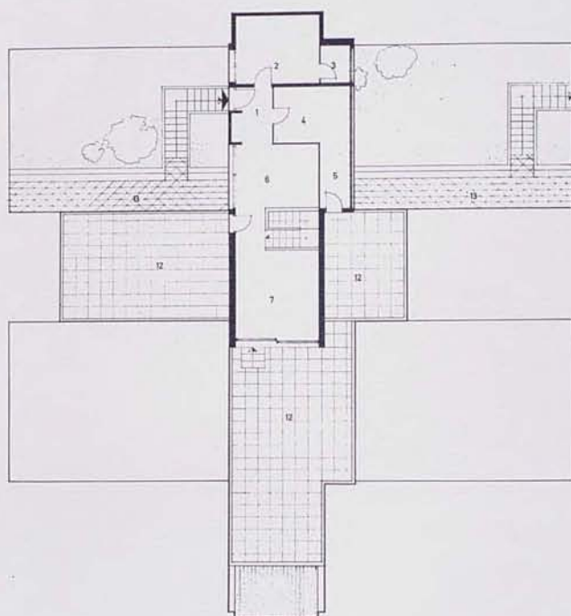
Planta piso de las viviendas tipo
