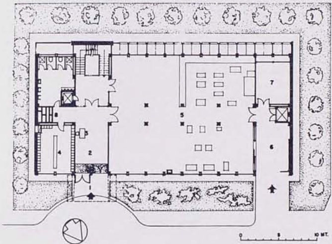
Planta baja de los laboratorios
