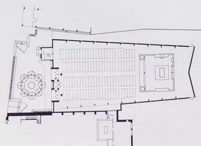
Planta
