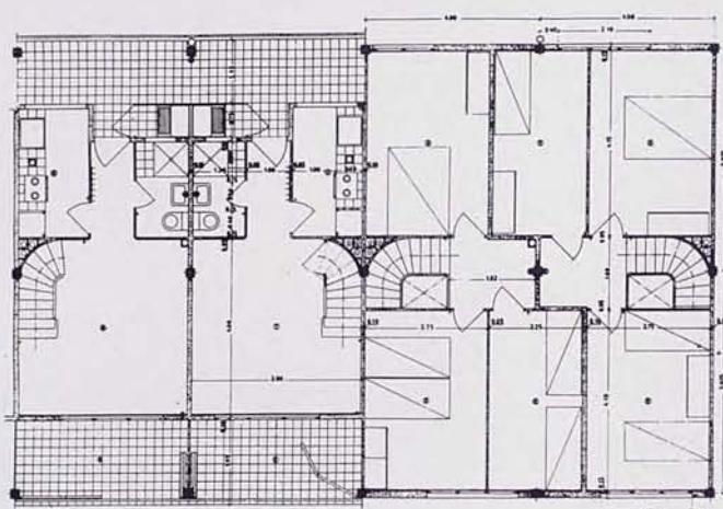
Planta acceso y piso de dos viviendas tipo
