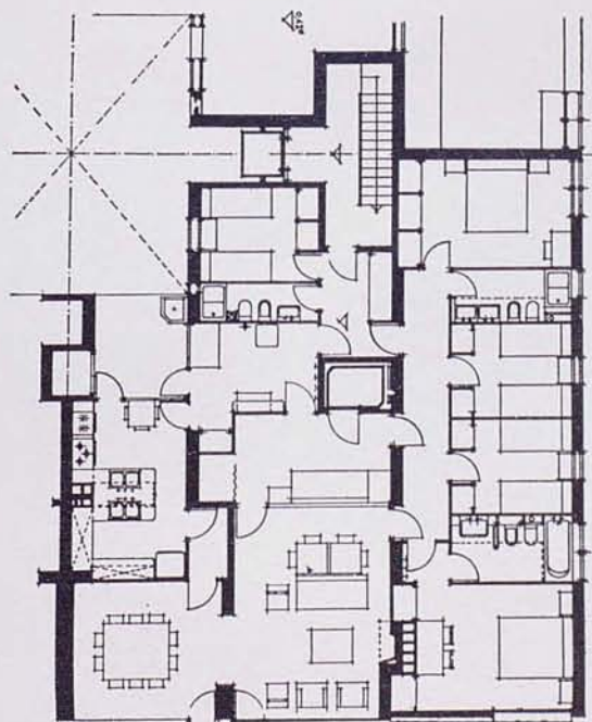
Plantas vivienda tipo
