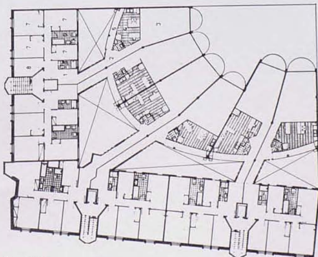
Planta tipo
