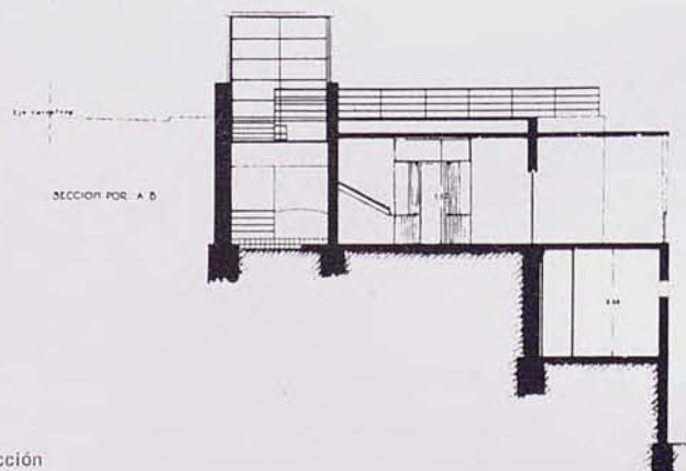
Sección
