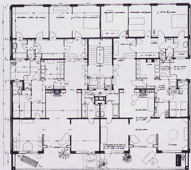
Planta tipo
