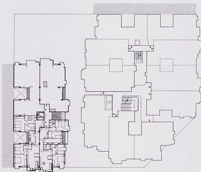
Planta general pisos tipo
