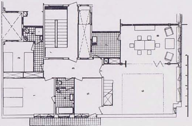
Planta inferior de la vivienda tipo
