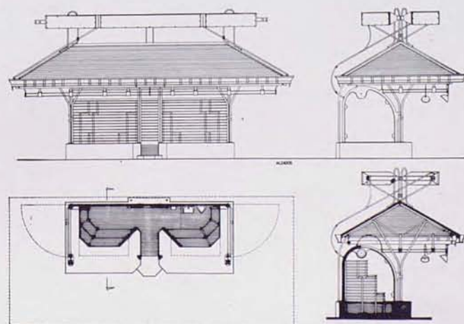
Alzados, Planta, Sección
