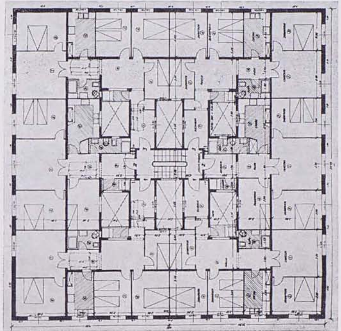
Planta tipo bloque Avda. Hospital Militar
