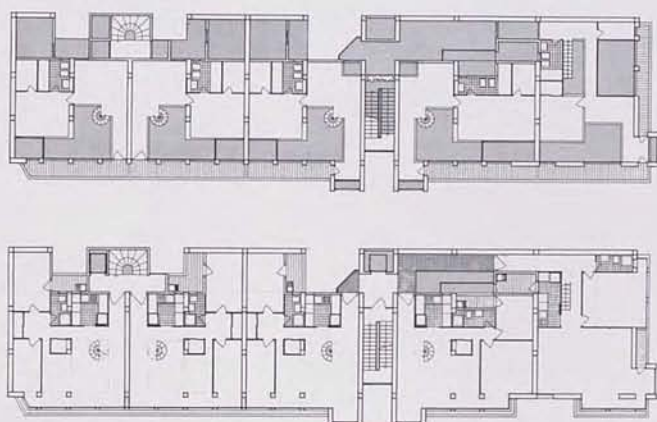
Plantas viviendas duplex
