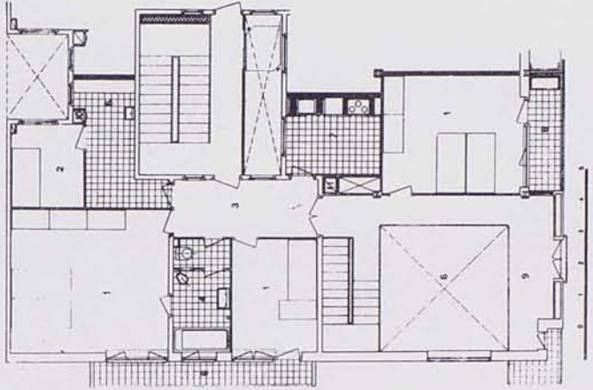
Planta superior de la vivienda tipo
