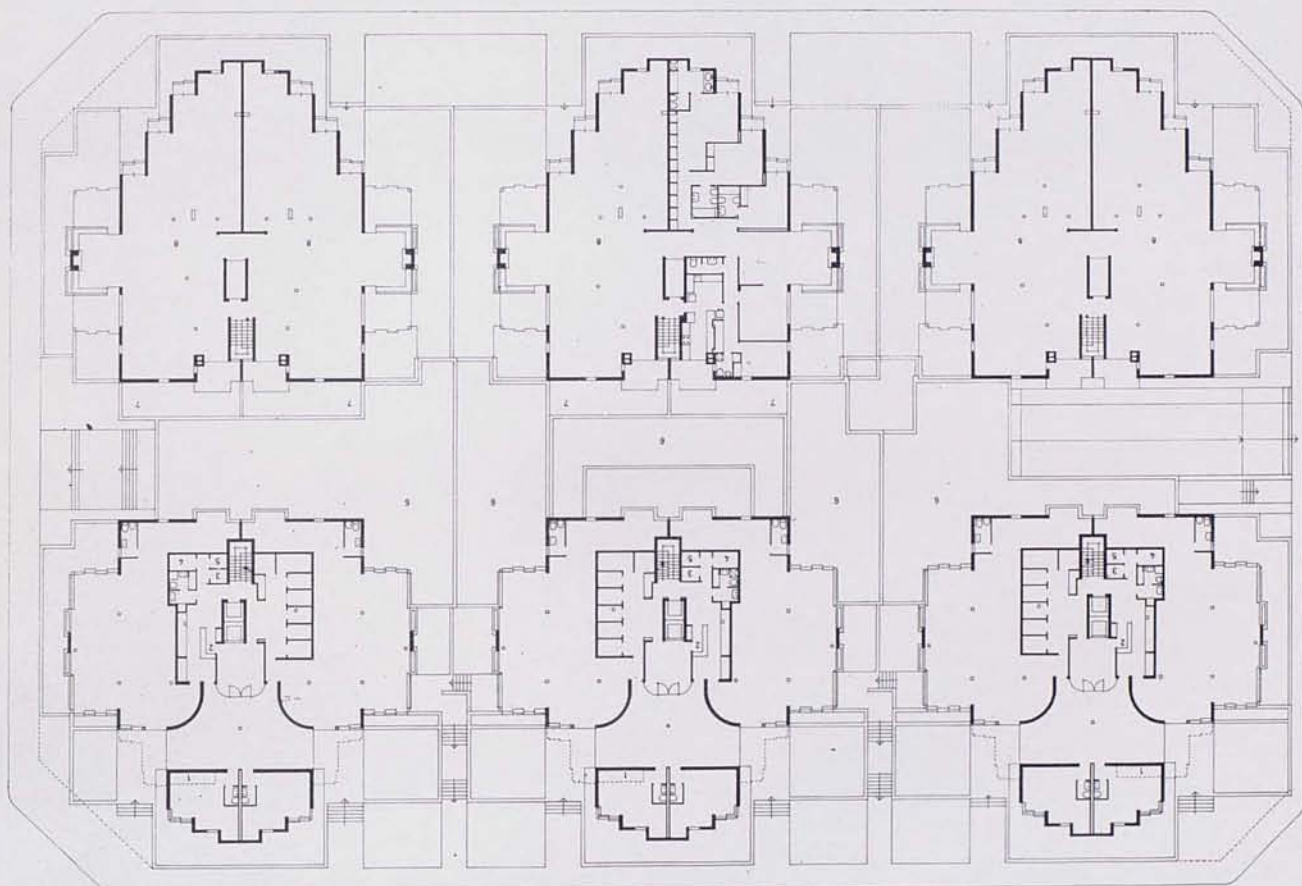
Planta general
