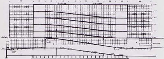
Sección longitudinal del almacén (Por la rampa de acceso a las plantas)
