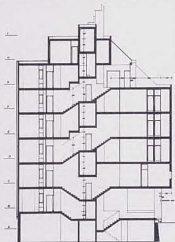
Sección
