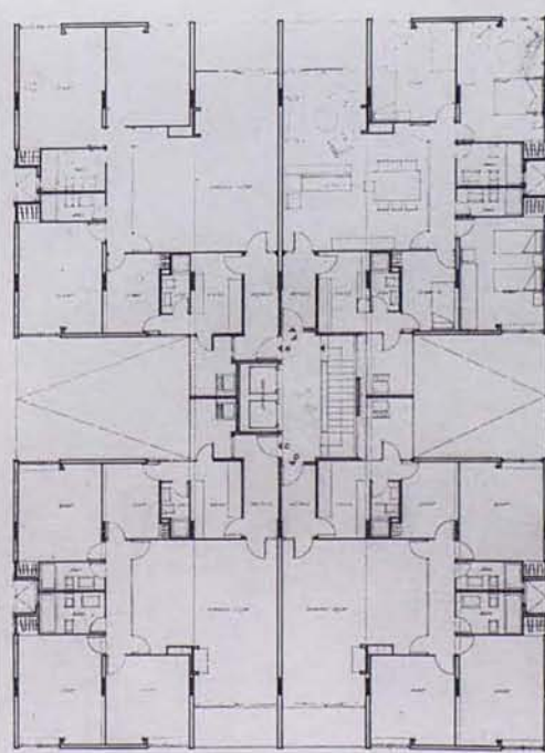
Planta tipo
