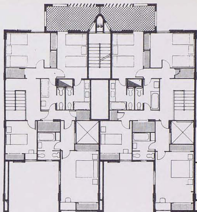
Plantas viviendas duplex
