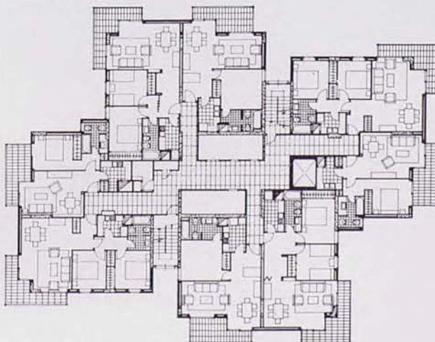
Plantas 4 a la 14
