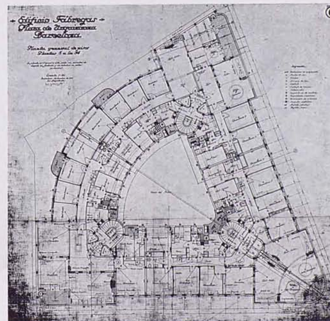
Planta tipo de los pisos 5 al 14
