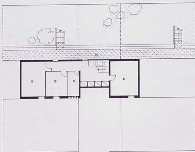
Planta baja de las viviendas tipo
