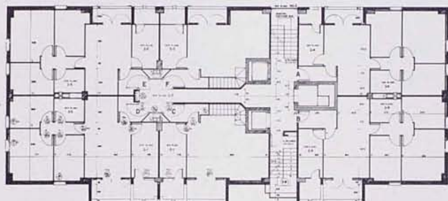
Plantas 1, 3, 5, 7.
