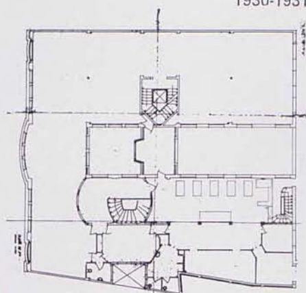
Planta piso
