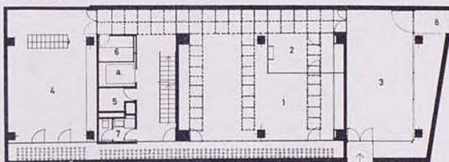
Planta sótano
