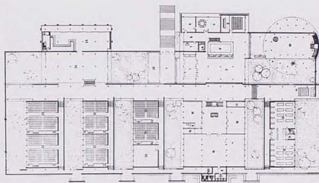
Planta baja
