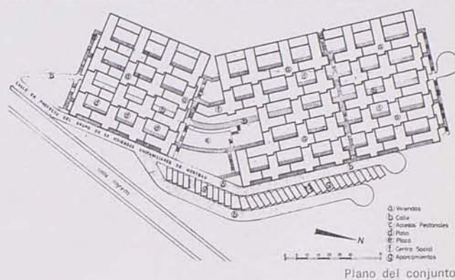
Plano del conjunto
