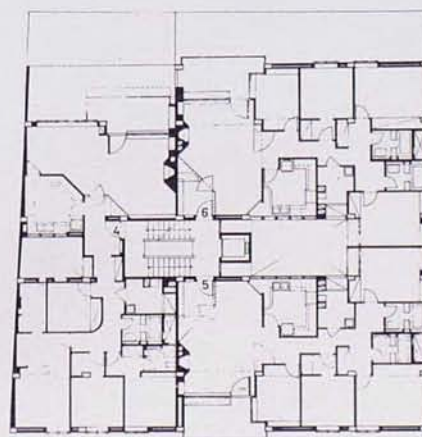
Planta 1.ª
