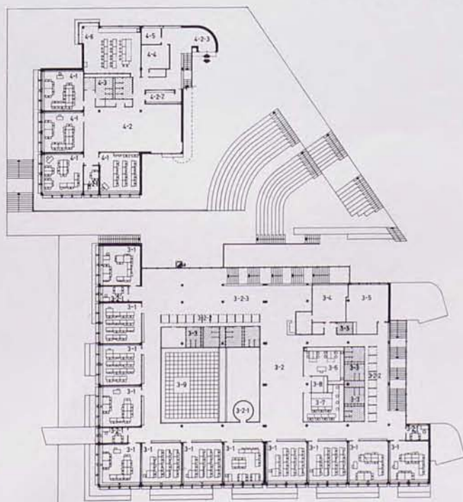
Plantas
