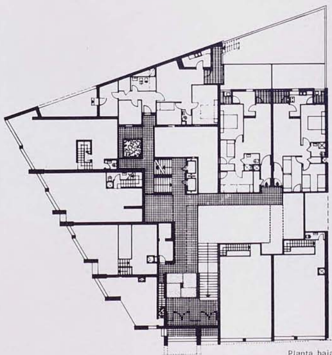
Planta baja
