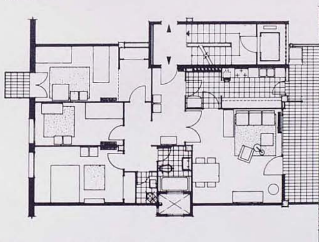
Planta viviendas tipo del bloque C
