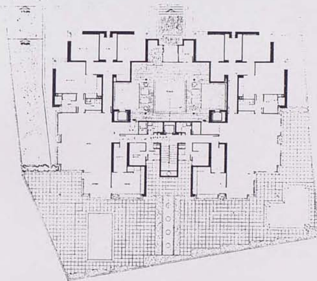
Planta entresuelo
