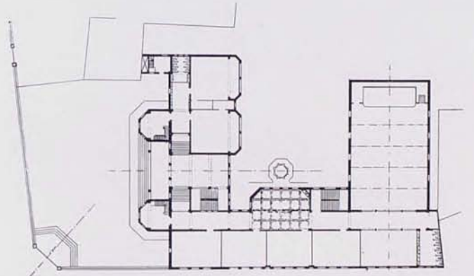
Planta baja
